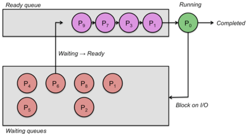
Figura: Escalonamento de processos.
