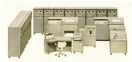
(b) B500
